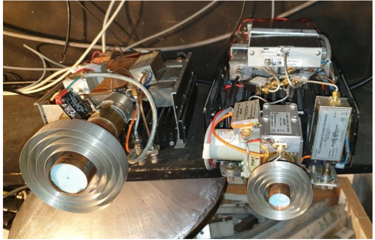
Systèmes pour EME à 5 et 10GHz, avec illuminateurs de parabole (Septum feed)
